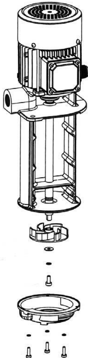
Pompa do Chłodziwa COLP 1-180T
