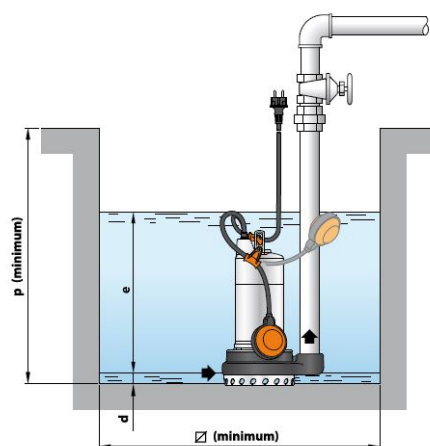
TYPOWA INSTALACJA
