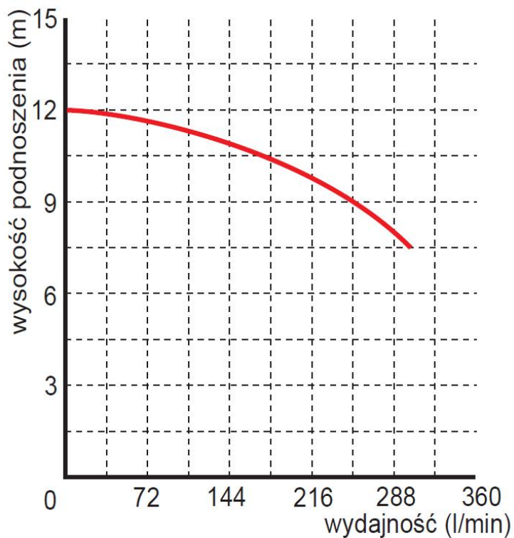
Wykres wydajności:
