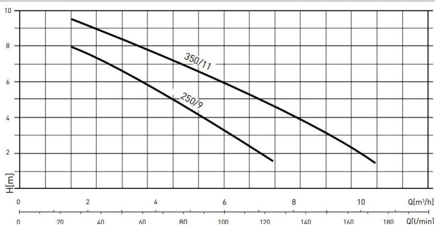
CHARAKTERYSTYKI POMP
