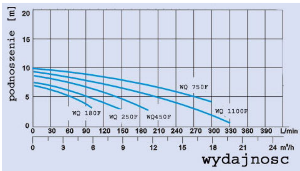
Wykres wydajności:
